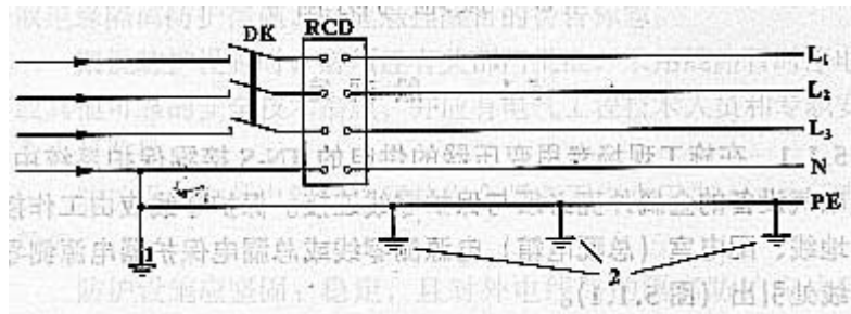
图 5.1.2 三相四线供电时局部 TN-S 接零保护系统保护零线引出示意
