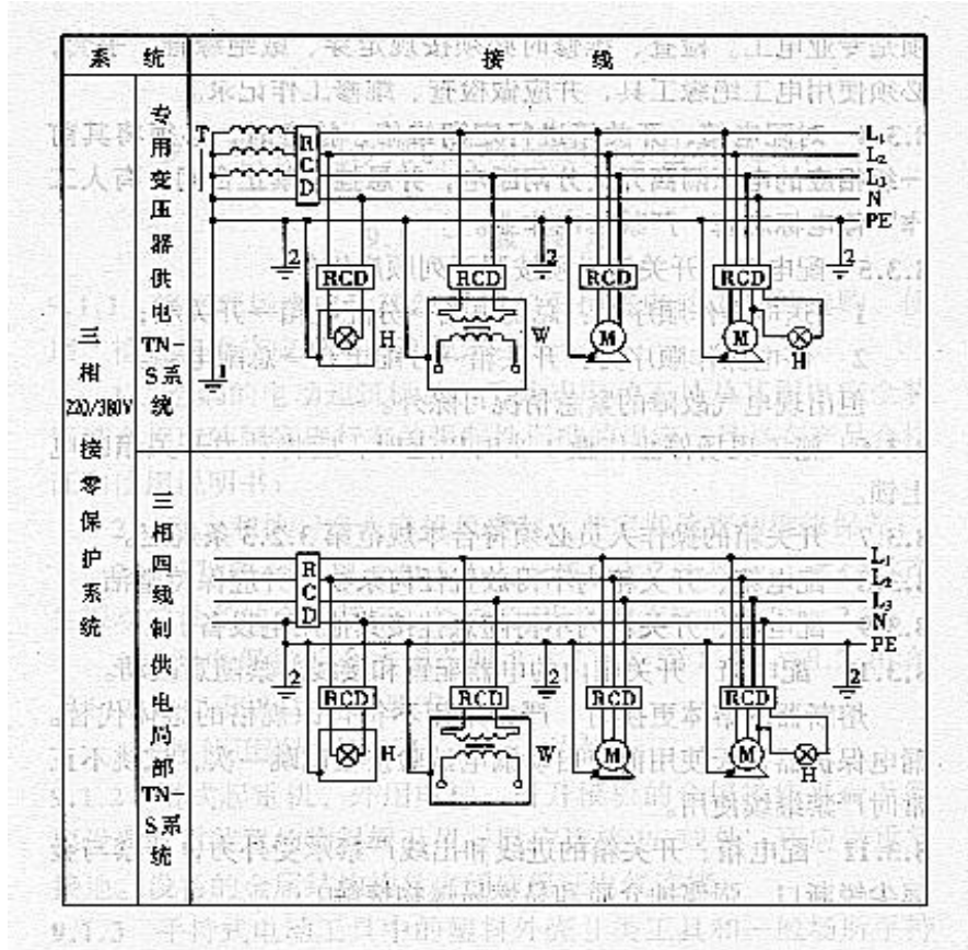
图 8. 2. 14 漏电保护器使用接线方法示意
